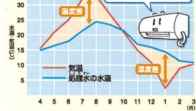
■処理水の水温と気温の比較
